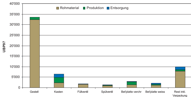
Abbildung 4: Umweltbelastung der verschiedenen Spülkastenkomponenten
